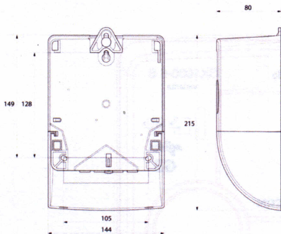
Slika 3. Nacrt brojila s izmjerama
