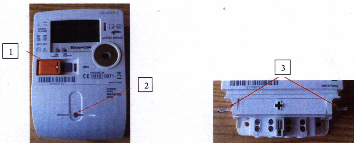
Slika 6. Slika brojila s označenim mjestima za ovjerne žigove i zaštitne plombe
