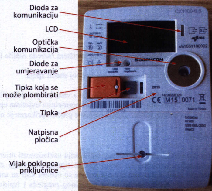
Slika 2. Izgled brojila
