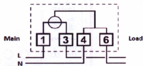
Slika 4. Shema spajanja
